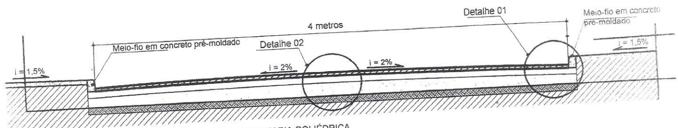
CORTE TRANSVERSAL DA PISTA DE ROLAMENTO - ALVENARIA POLIÉDRICA
