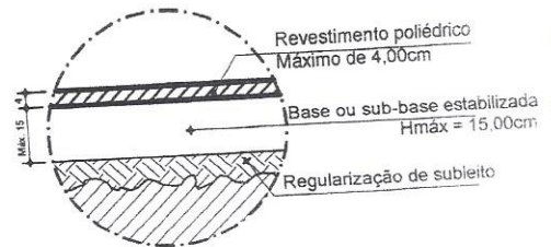
DETALHE 02 - CORTE CAMADAS PMF
